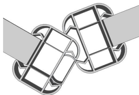
Figuur 23 en 24: voorbeelden van schuine hoeken
