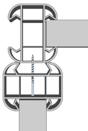
Figuur 20: hoek 90° mogelijkheid 2
