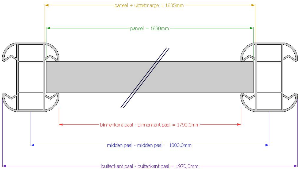
Figuur 1: afmetingen
