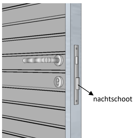
Figuur 36: detail slot tuindeur
